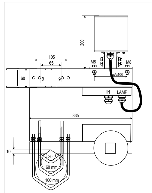
CEL-50-230-CST Obstacle Light dimensions
