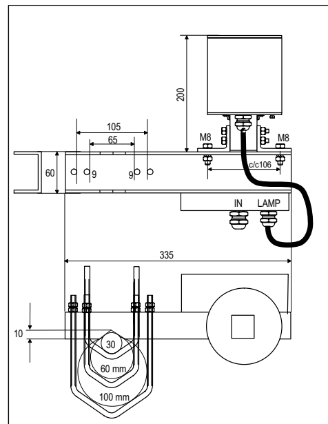
CEL-50-230-CST Obstacle Light dimensions
